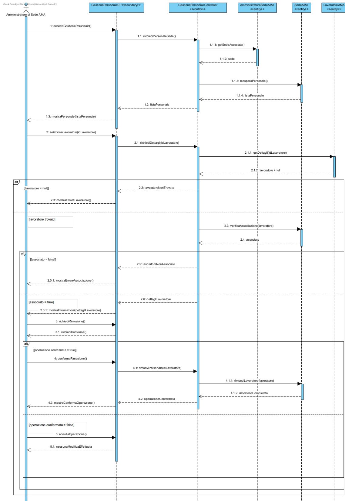
Figura 42: Sequence Diagram — Rimuovere personale
