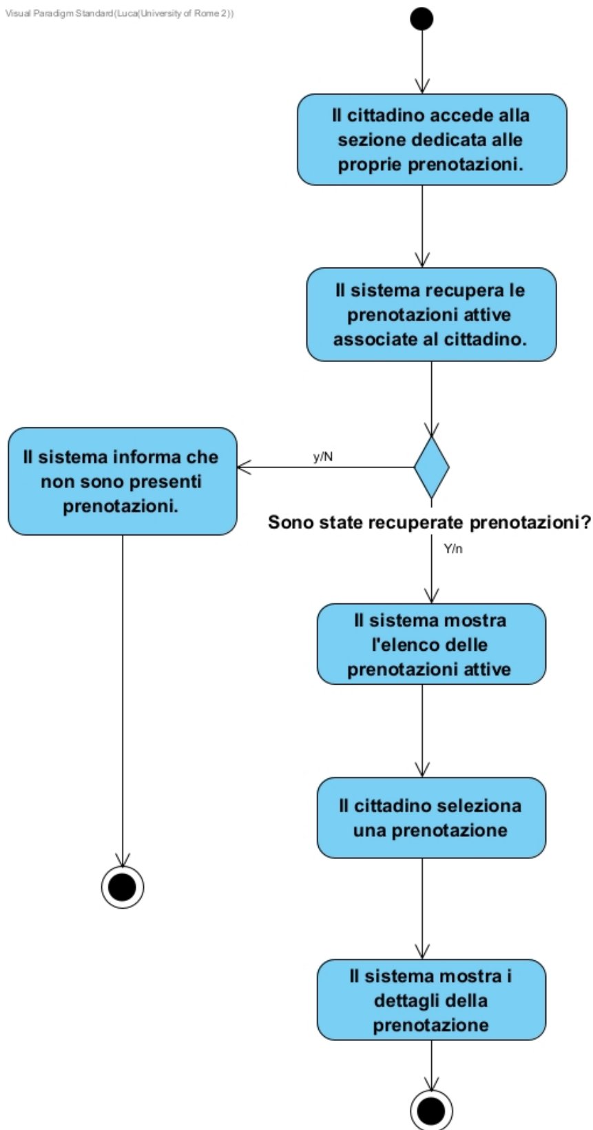
Figura 12: Activity Diagram — Visualizzare prenotazioni attive
