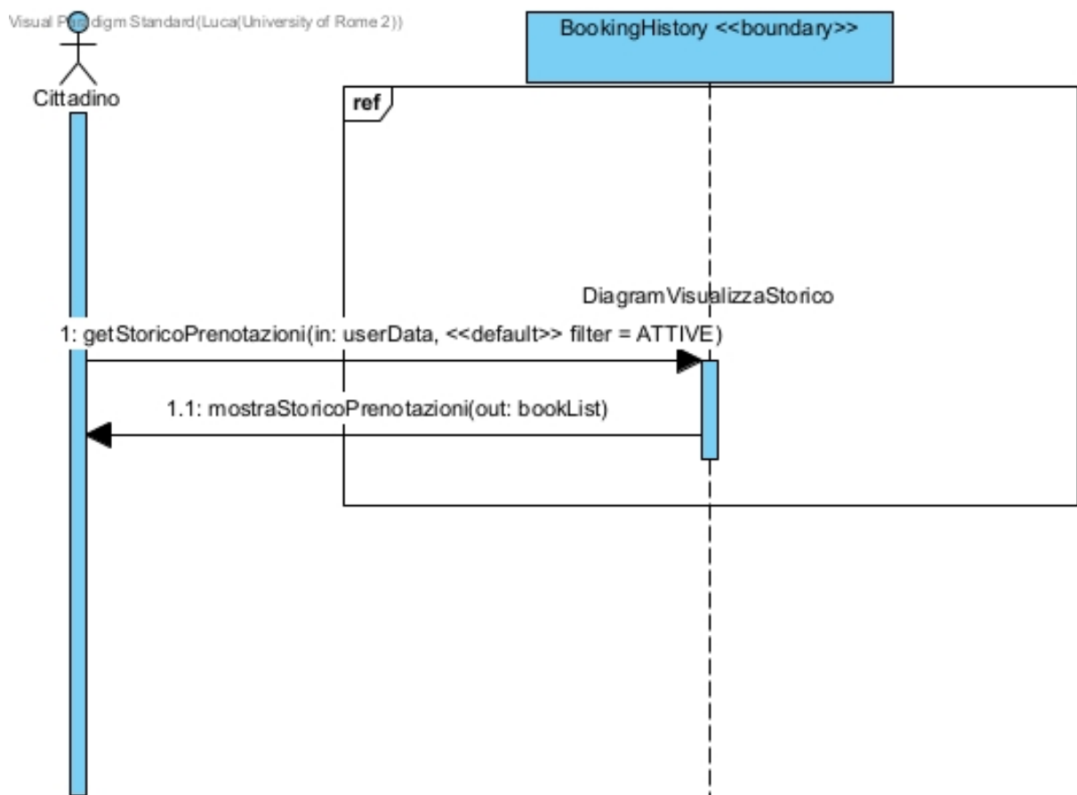
Figura 27: Sequence Diagram — Visualizzare prenotazioni attive
