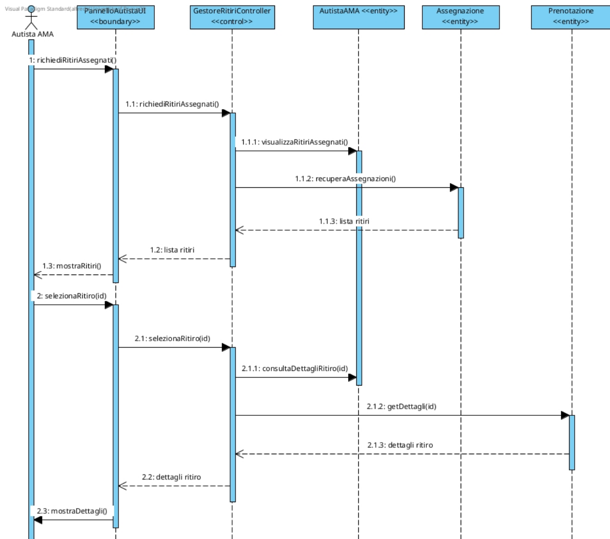
Figura 31: Sequence Diagram — Visualizzare ritiri assegnati
