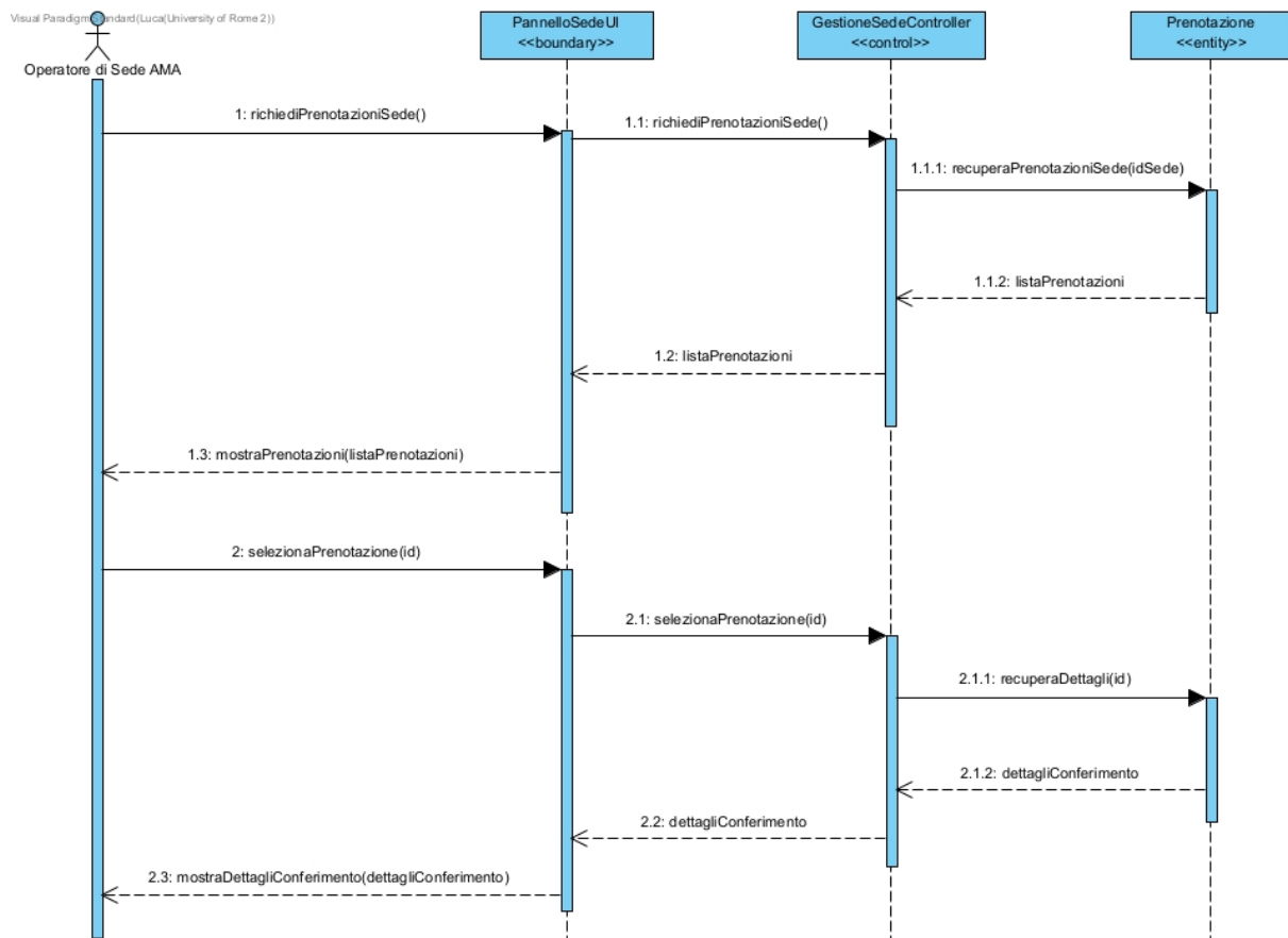
Figura 34: Sequence Diagram — Visualizzare prenotazioni della sede
