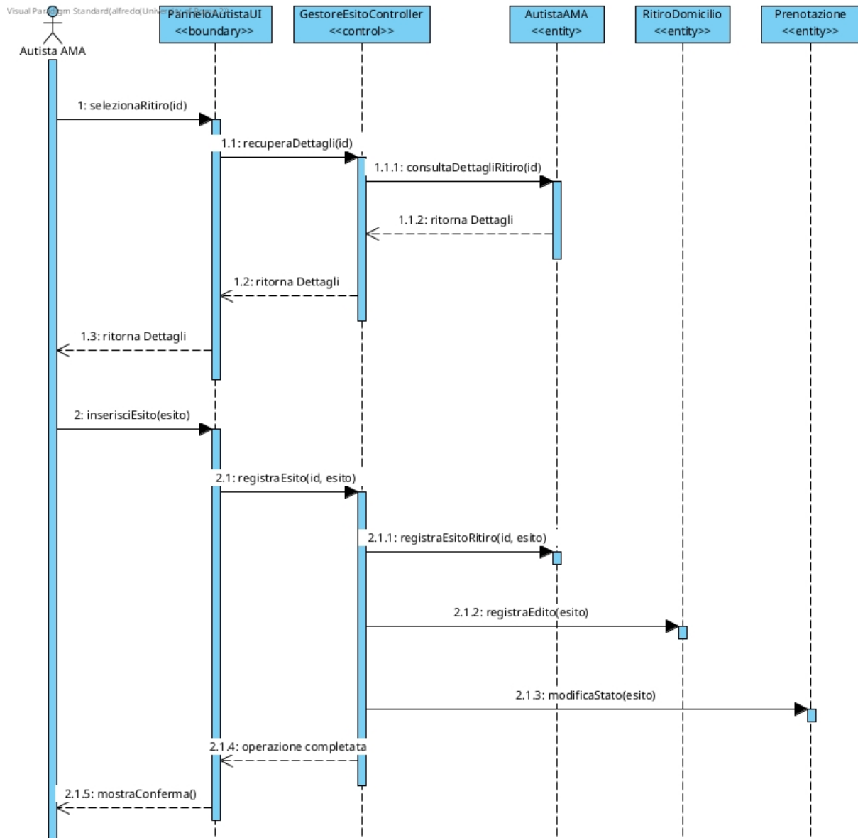
Figura 32: Sequence Diagram — Registrare esito del ritiro
