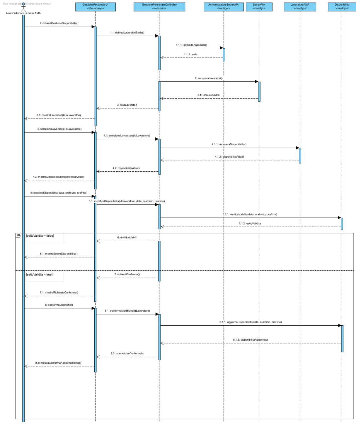
Figura 38: Sequence Diagram — Gestire disponibilità dei lavoratori
