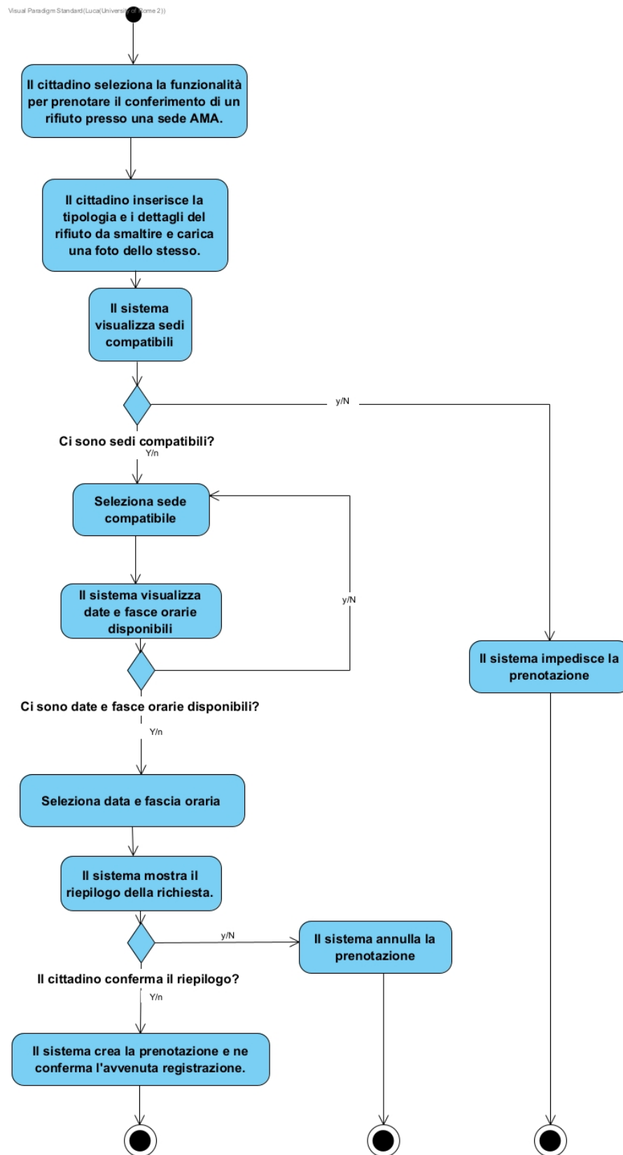
Figura 11: Activity Diagram — Prenotare conferimento in sede
