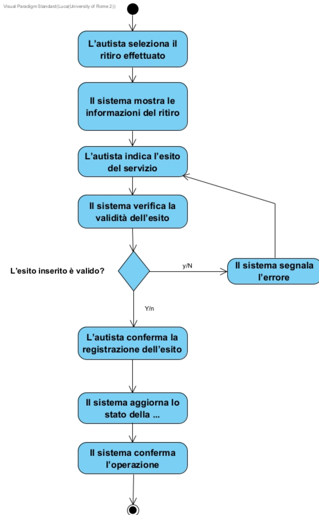
Figura 15: Activity Diagram — Registrare esito del ritiro (Autista)
