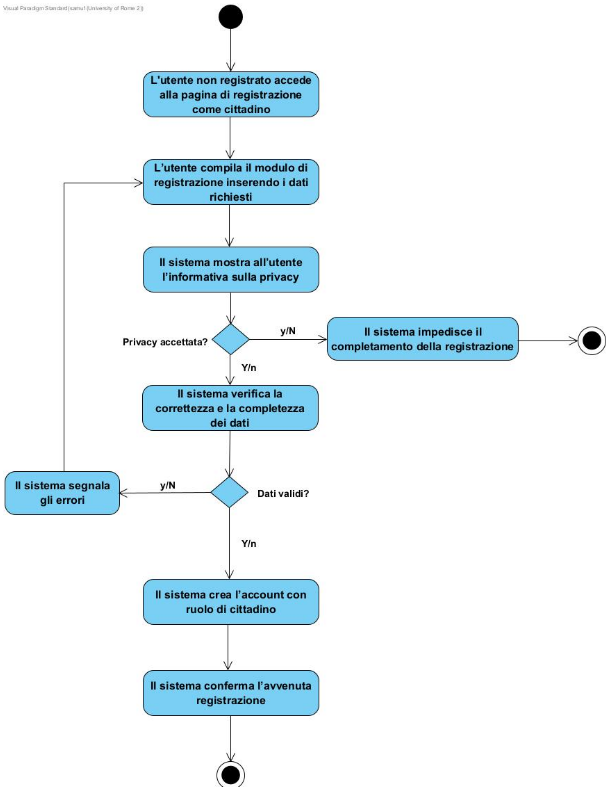
Figura 7: Activity Diagram — Registrarsi come cittadino
