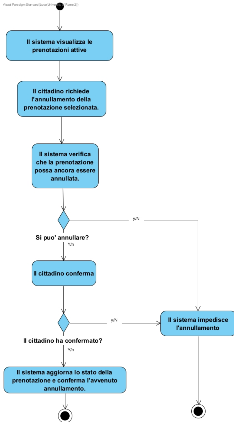
Figura 13: Activity Diagram — Annullare prenotazione
