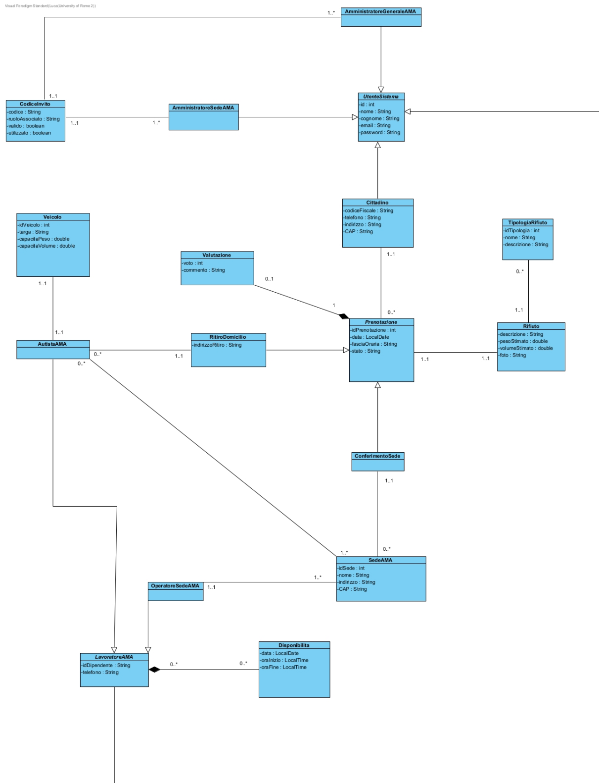
Figura 45: Class Diagram — Versione Unrefined (Modello di Dominio)
