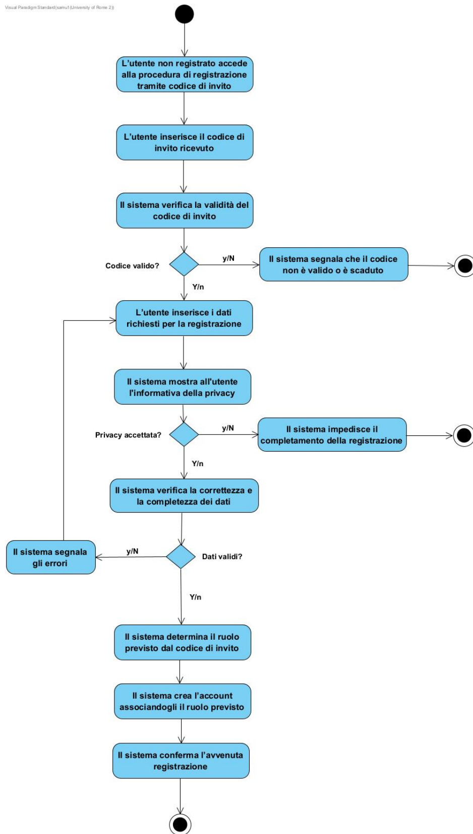
Figura 8: Activity Diagram — Registrarsi tramite codice di invito
