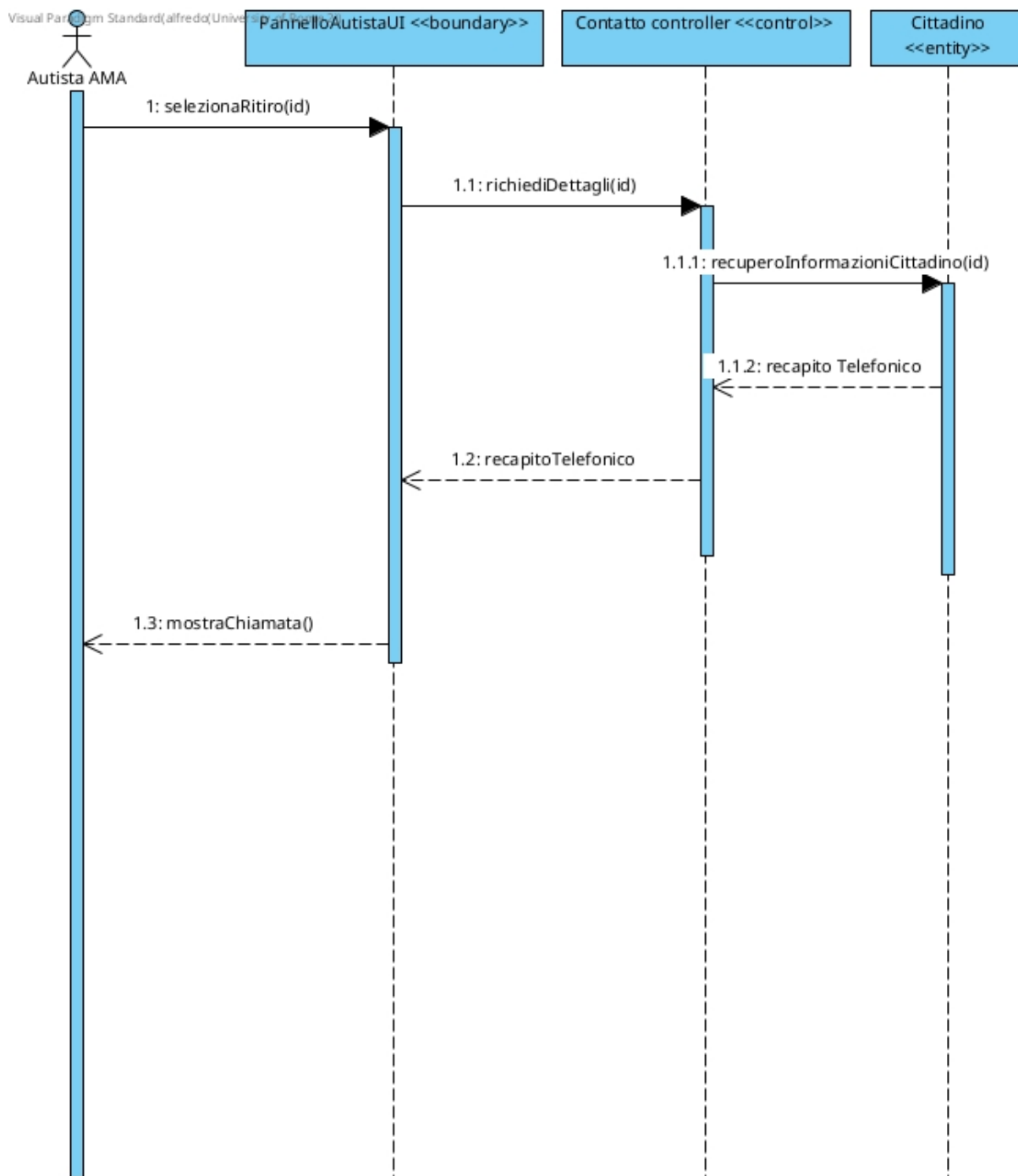
Figura 33: Sequence Diagram — Chiamare cittadino
