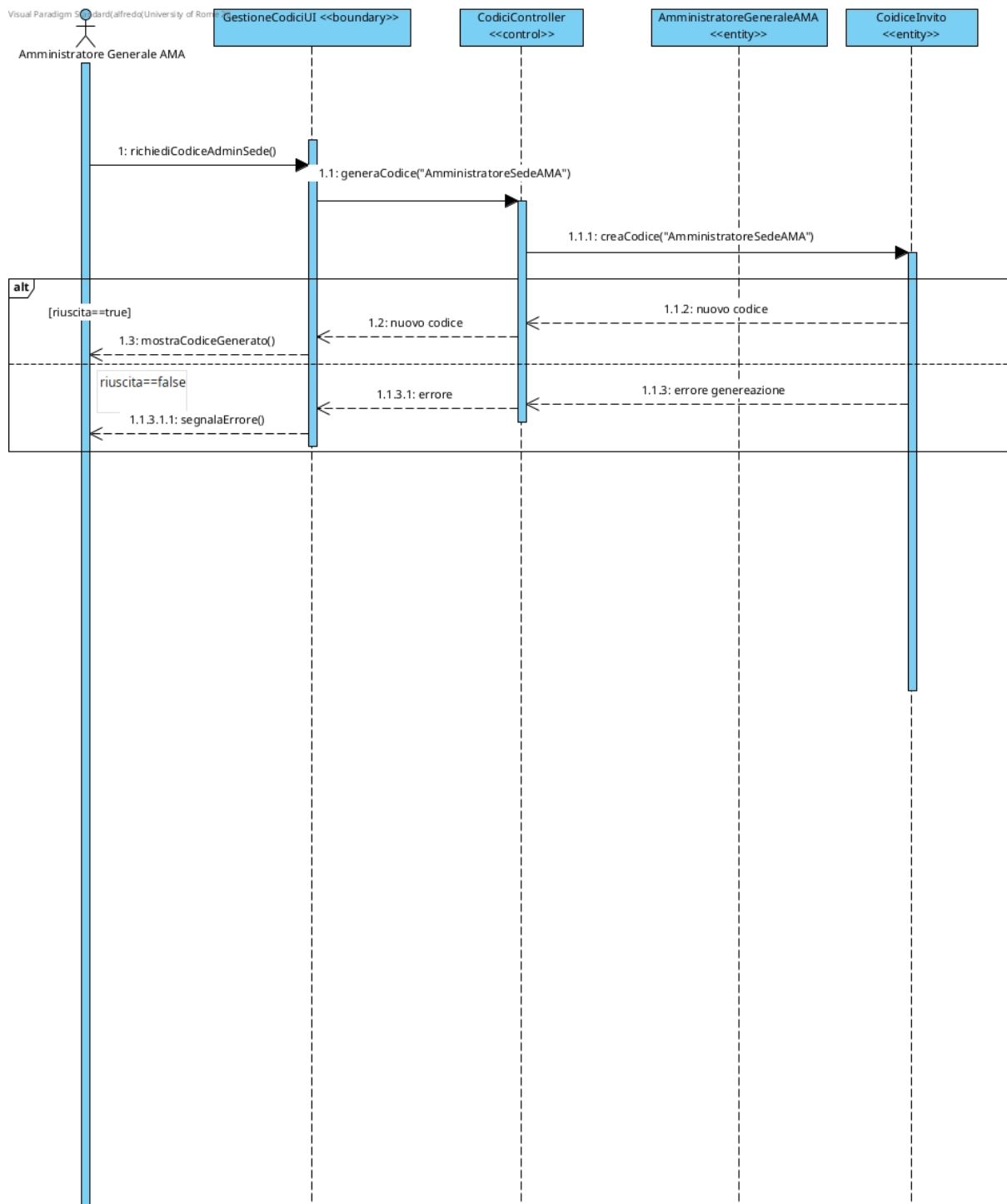
Figura 43: Sequence Diagram — Generare codice amministratore di sede
