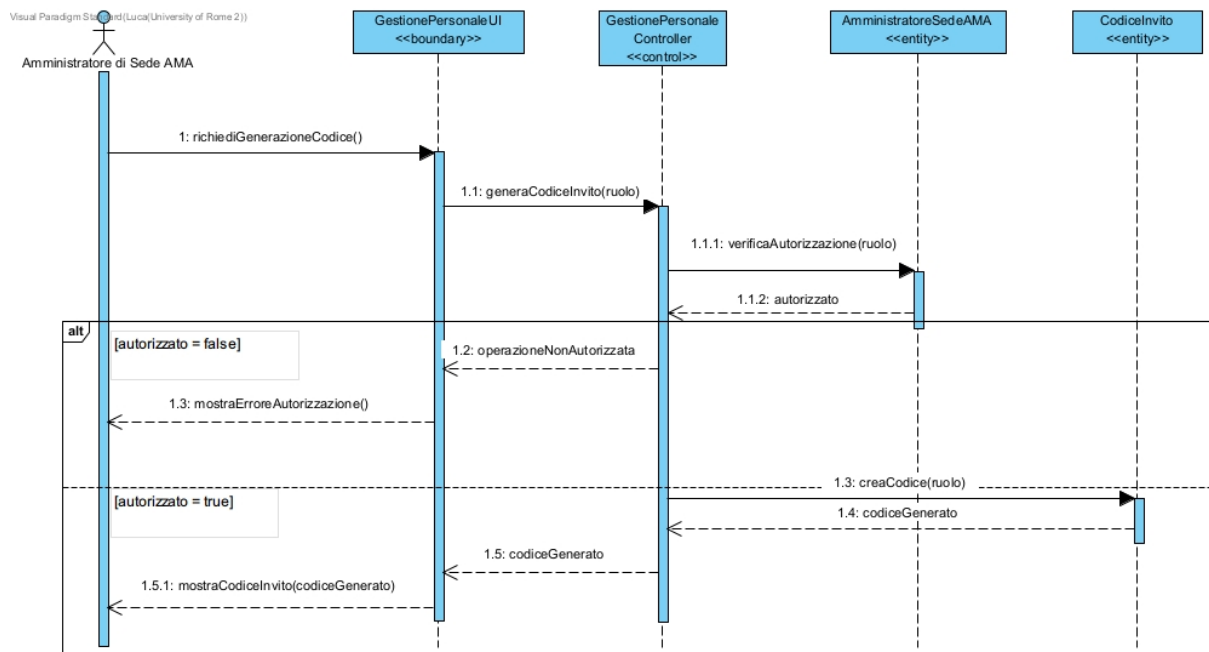
Figura 37: Sequence Diagram — Generare codice invito
