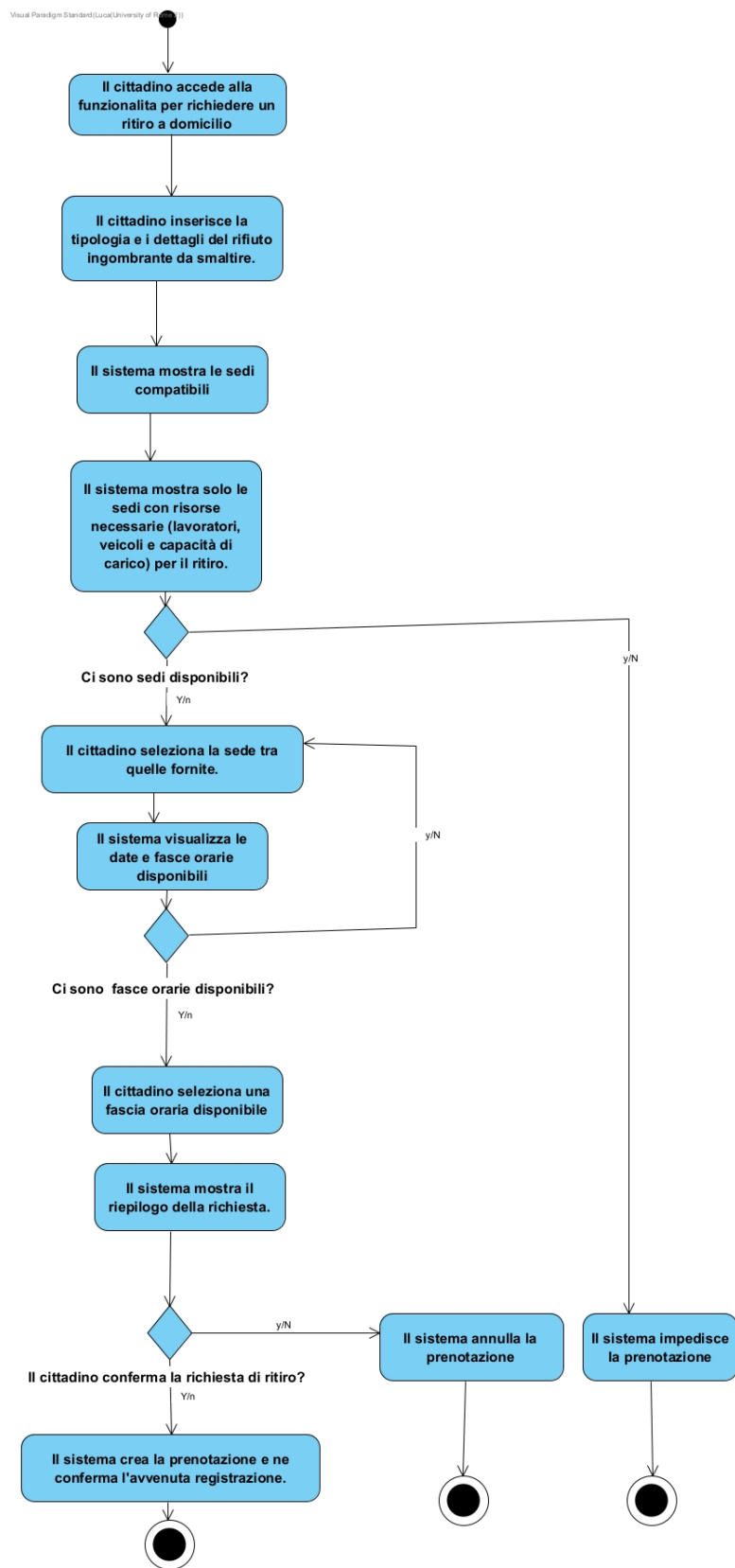
Figura 10: Activity Diagram — Richiesta ritiro a domicilio
