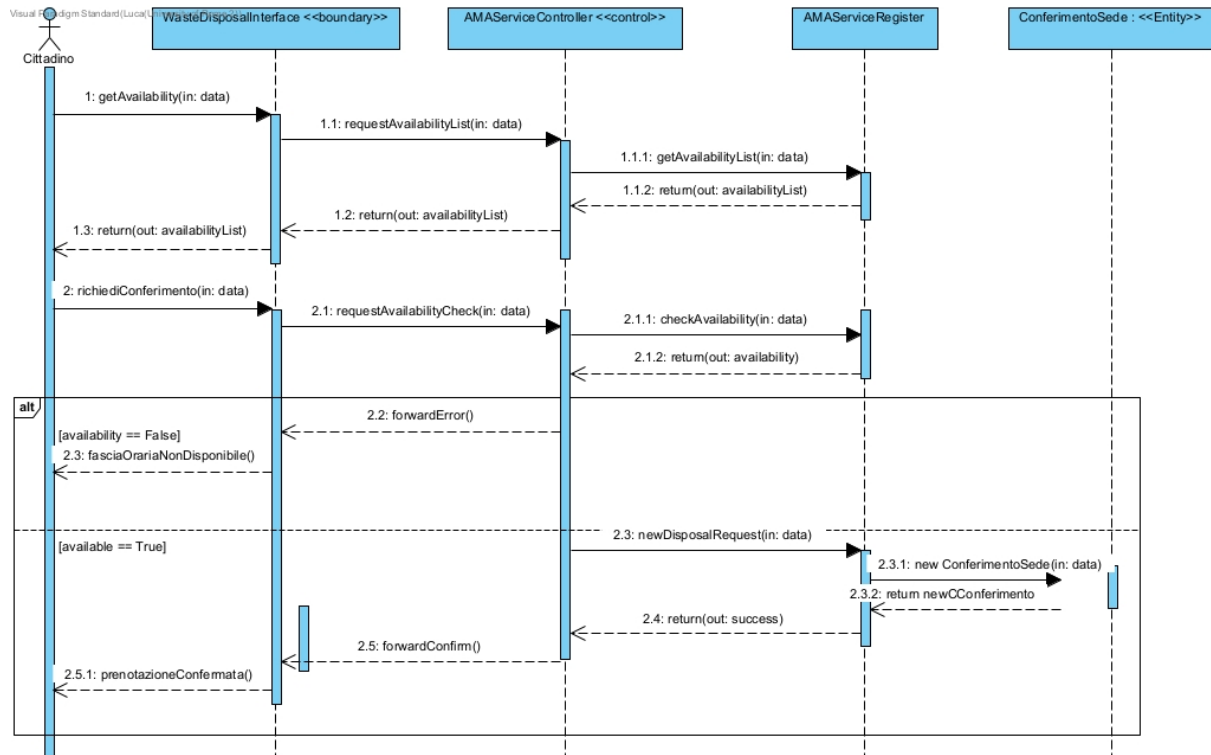
Figura 26: Sequence Diagram — Prenotare conferimento presso sede AMA
